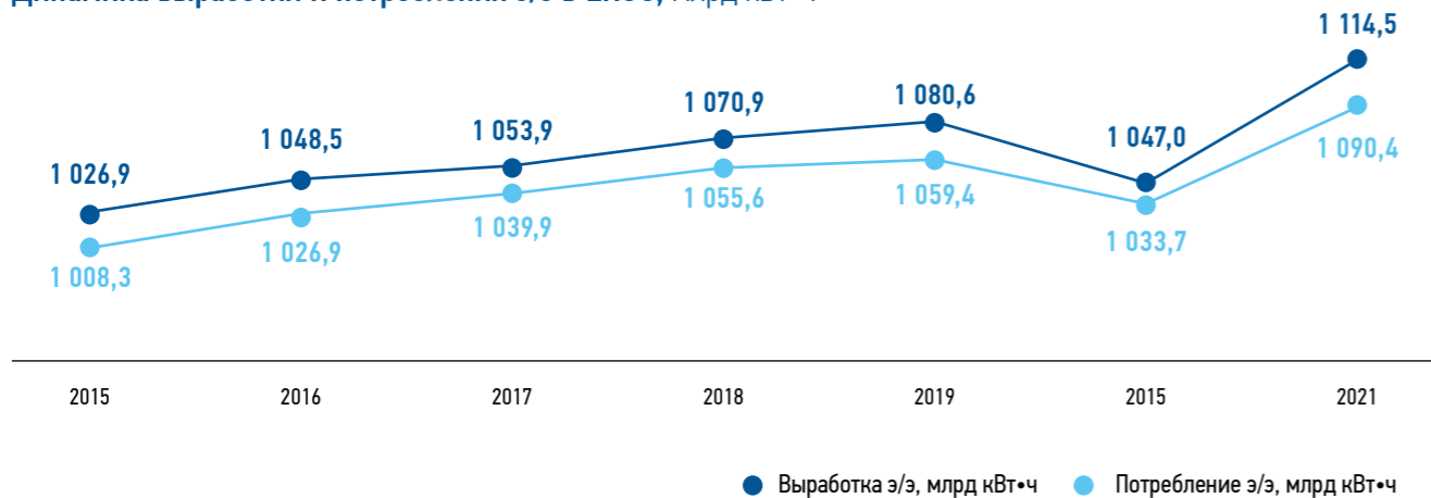
Динамика выработки и потребления э/э в ЕНЭС, млрд кВт•ч
